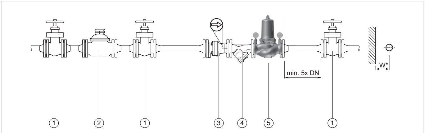
Abb. 1 Beispiel für den standardmäßigen Einbau für Druckminderer
