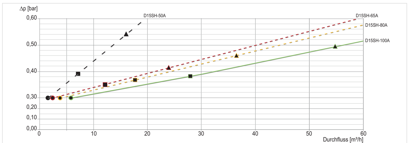
Abb. 2 Druckabfall innerhalb des Ventils für Nennweite DN50 bis DN100.
