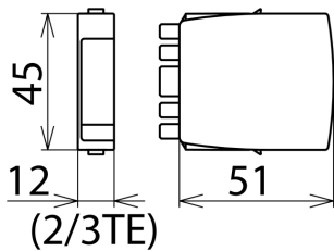
Maßbild BXT ML4 BD EX 24
