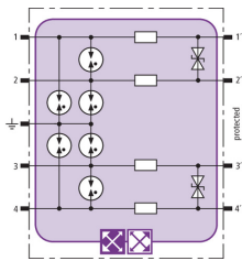
PrinzipschaltbildBXT ML4 BD EX 24
