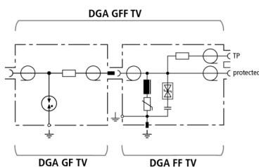
Prinzipschaltbild DGA GFF TV – kombiniert aus DGA GF TV und DGA FF TV
