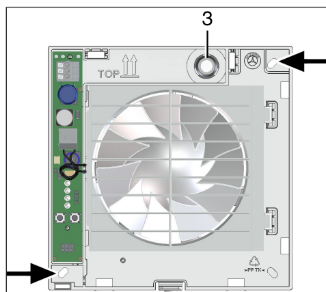
3 Cable grommet
