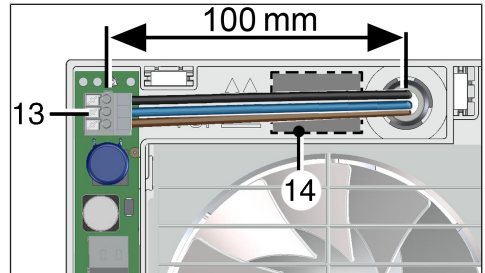
13 Federklemme
