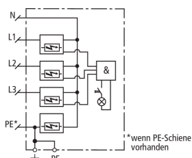
Prinzipschaltbild DV ZP TT 255
