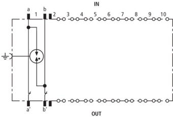
Prinzipschaltbild DRL 10 B 180
