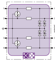
Principalschaltbild BXT ML4 BE 24
