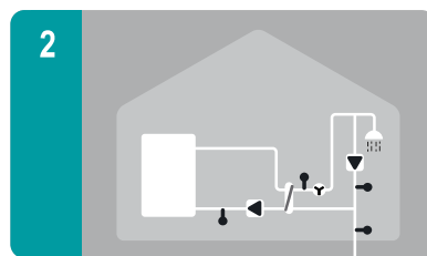
Fertigung von Brauchwasser mit Zirkulation
