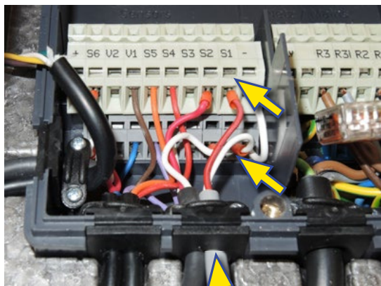
Abb. 6: Anschließen der Zirkulationstemperatursonde.
