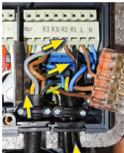
Abb. 7: Anschluss des Umwälzpumpe.
