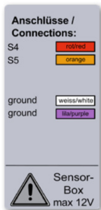
Abb. 4: Anschluss der Fühler an die Sensor Box
