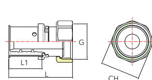
ÜBERGANGSPRESSVERSCHRAUBUNG FLACHDICHTEND / RACCORD À SERTIR ET ÉCROU TOURNANT JOINT PLAT
