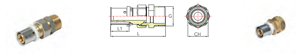
PRESSVERSCHRAUBUNG MIT AG KONISCH / RACCORD À SERTIR MÂLE ET ÉCROU TOURNANT CONIQUE
