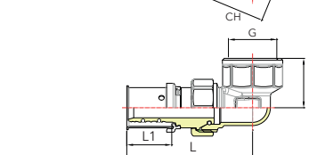
WINKELVERSCHRAUBUNG 90° MIT IG KONISCH / ÉCROU TOURNANT ET COUDE 90° FEMELLE CONIQUE
