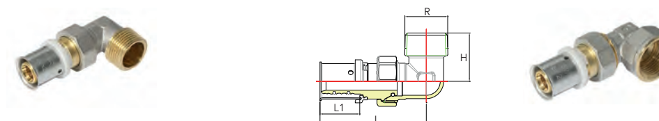
WINKELVERSCHRAUBUNG 90° MIT AG KONISCH / ÉCROU TOURNANT ET COUDE 90° MÂLE CONIQUE
