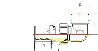
WINKELVERSCHRAUBUNG 90° MIT AG KONISCH / ÉCROU TOURNANT ET COUDE 90° MÂLE CONIQUE
