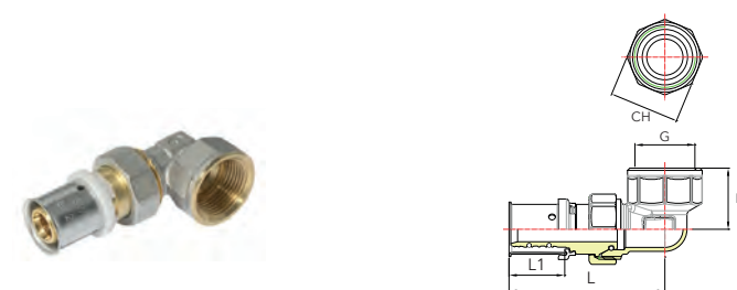
WINKELVERSCHRAUBUNG 90° MIT IG KONISCH / ÉCROU TOURNANT ET COUDE 90° FEMELLE CONIQUE
