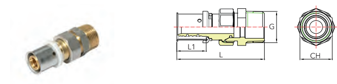
PRESSVERSCHRAUBUNG MIT AG KONISCH / RACCORD À SERTIR MÂLE ET ÉCROU TOURNANT CONIQUE
