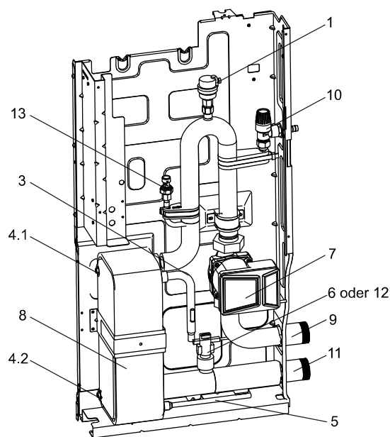
8–16-kW-Gerät ohne Reserveheizer
