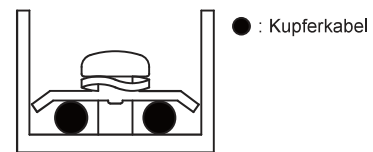
Korrekte Stromversorgungsverkabelung
