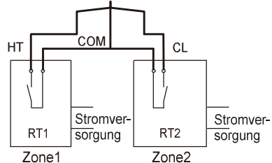
Methode C (Zwei-Zonen- Steuerung)
