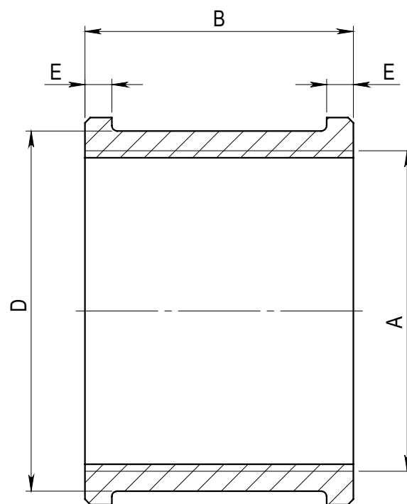
A-A
