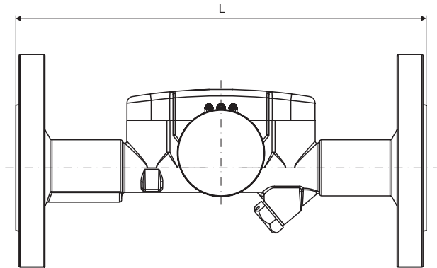
Abmessung Durchflusssensor mit Flanchanschluss
