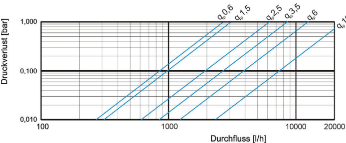
Druckverlustkurve
