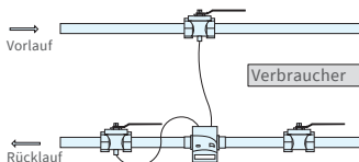
Symmetrischer Fühlereinbau bei zelsius C5-IUF
