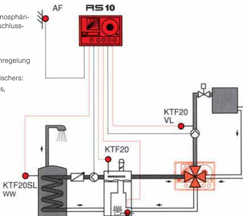
Einbaulage der Regelstation
