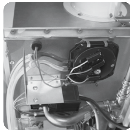
Druckwächter DL, mit D-Clip an Heizkessel befestigt
