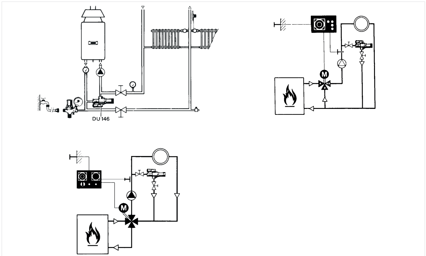
Abb. 1 DU146 in Heizkreisen mit Kessel, in Heizsystemen mit 3-Wege- oder 4-Wege-Mischventil.
