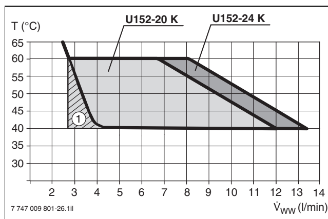
Bild 27 Diagramm für eine Kaltwasser-Einlaufftemperatur von +15 °C
