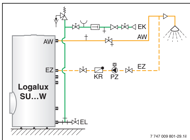
Bild 29 Variante einer Zirkulationsleitung für die Warmwasserspeicher Logalux SU...W
