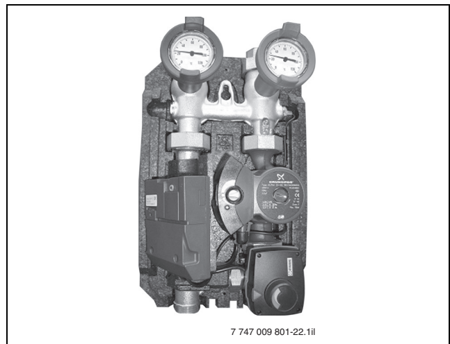
Bild 22 Heizkreis-Schnellmontage-Set mit integriertem Mischermodul MM10
