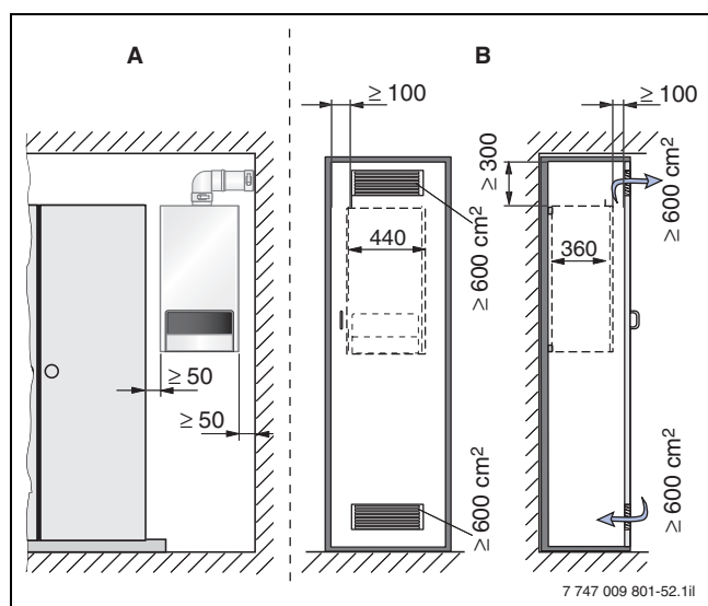
Bild 52 Empfohlene seitliche Mindestabstände für Wartungen am U152 (Maße in mm); Buderus-Umbauschrank V60 → Seite 55
