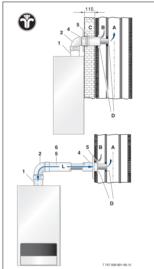
Bild 90 Montagevariante mit dem Bausatz LAS-K für U152 (Maße in mm); maximal zulässige gestreckte Baulänge L der Abgasleitung → Tabelle 39, Bauteile → Seite 99
