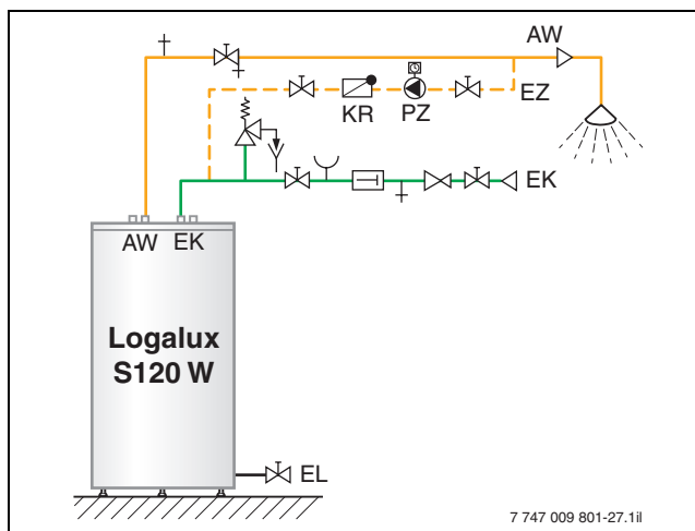
Bild 28 Variante einer Zirkulationsleitung für den Warmwasserspeicher Logalux S120 W
