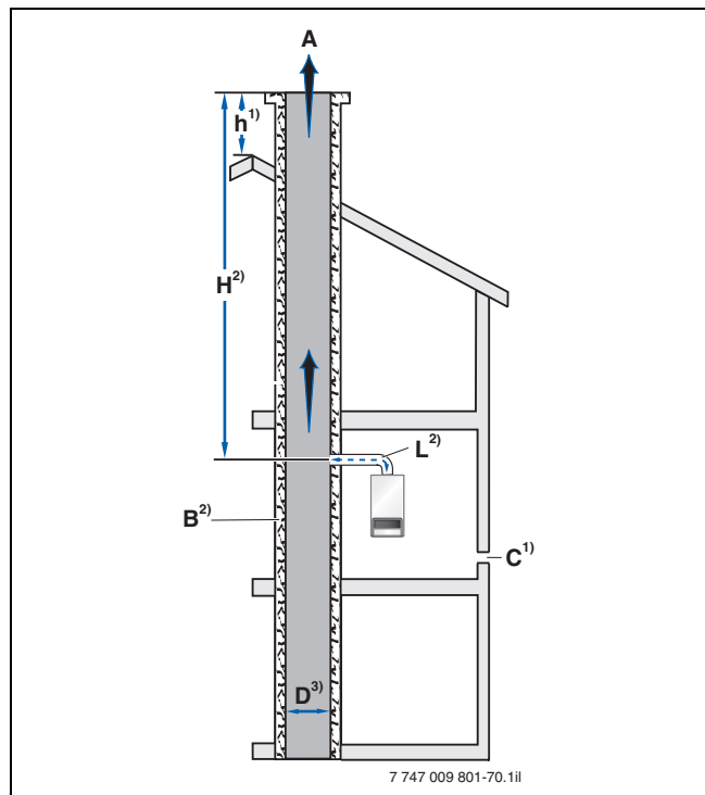
Bild 70 Normen für den Anschluss eines U154 an eine eigene Abgasanlage
