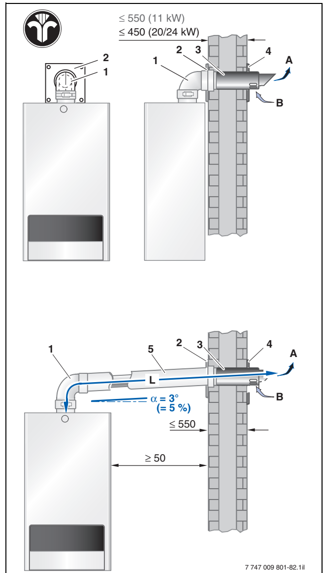
Bild 82 Montagevarianten der Luft-Abgas-Leitung waagrecht nach hinten (WH) oder zur Seite (WS) mit dem Bausatz WH/WS für U152 (Maße in mm); maximal zulässige gestreckte Baulänge L der Abgasleitung → Tabelle 32, Bauteile → Seite 90
