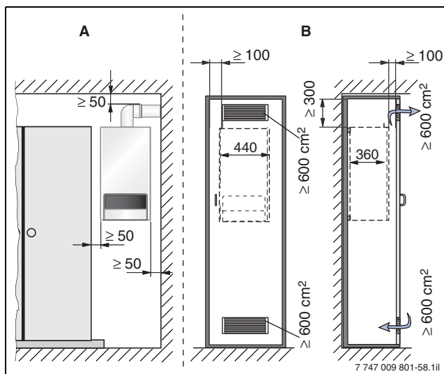
Bild 58 Sicherheitsabstand vom 1-wandigen Abgasrohr zur Decke und empfohlene seitliche Mindestabstände für Wartungen am U154 (Maße in mm); Buderus-Umbauschrank V60 → Seite 55
