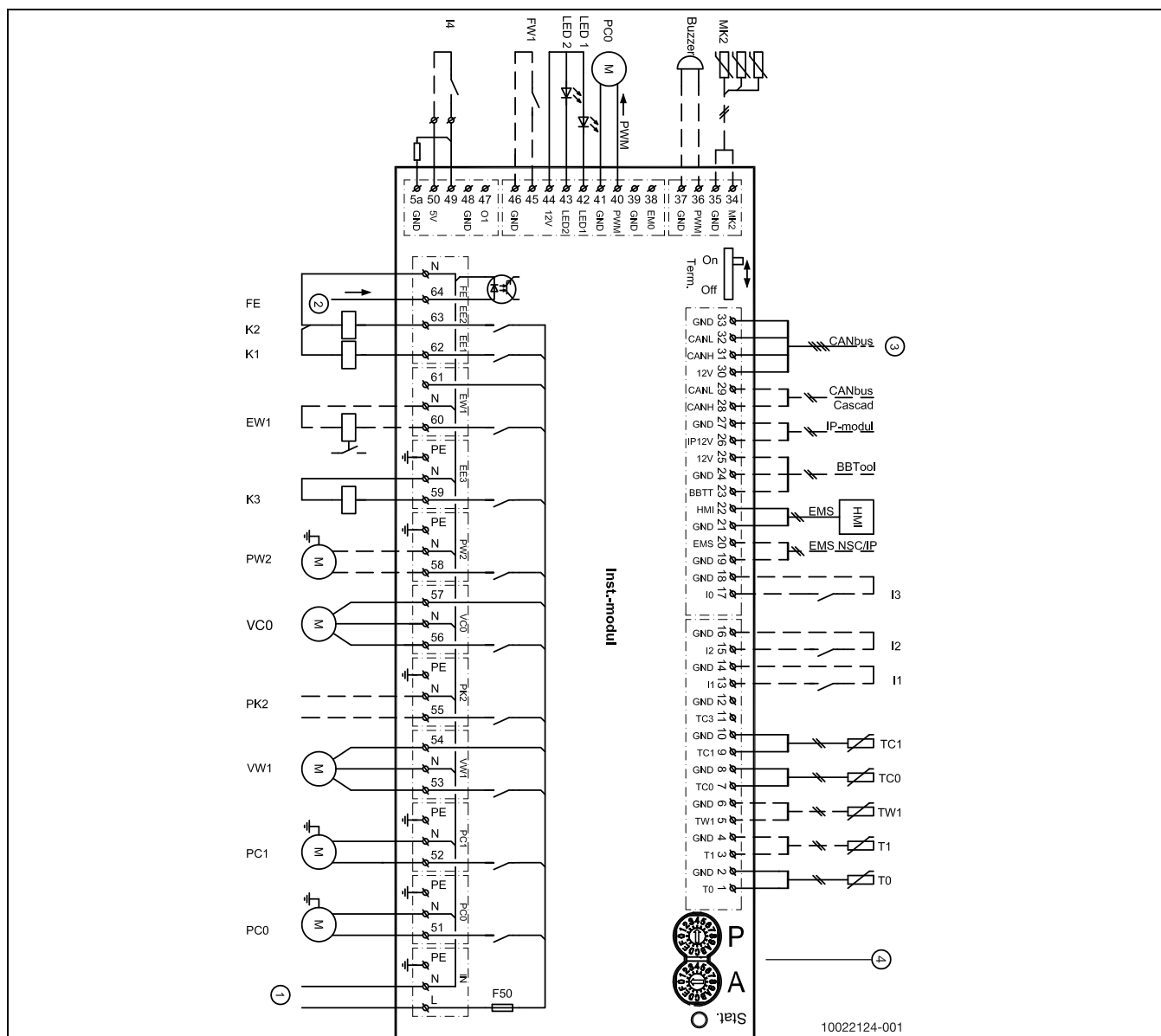
Bild 51 Schaltplan Installationsmodul
