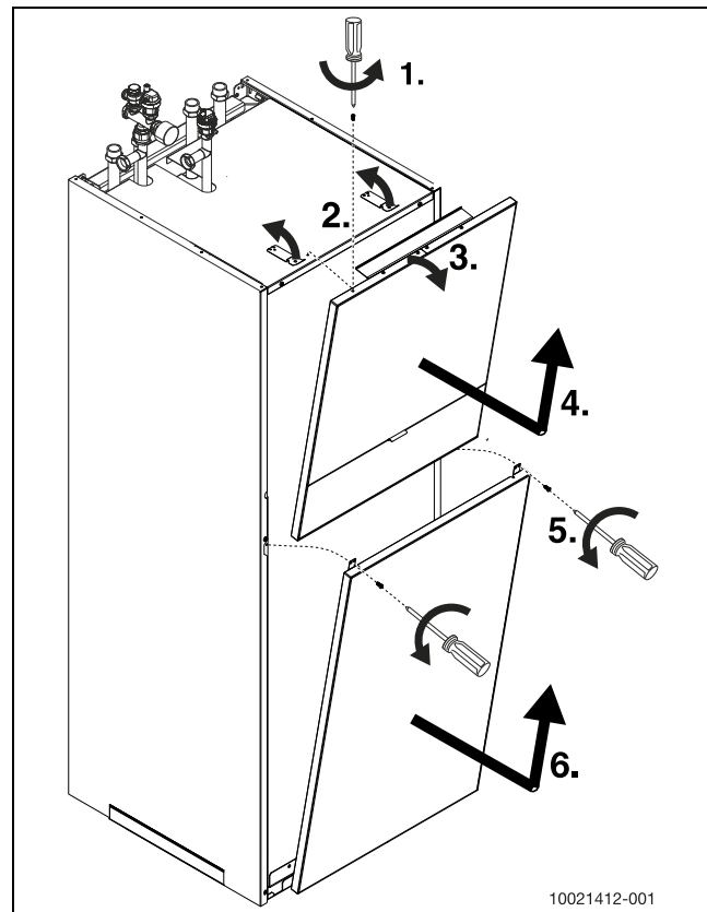
Bild 9 Abdeckungen entfernen
