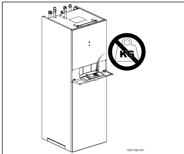
Bild 22 Regelgerät
