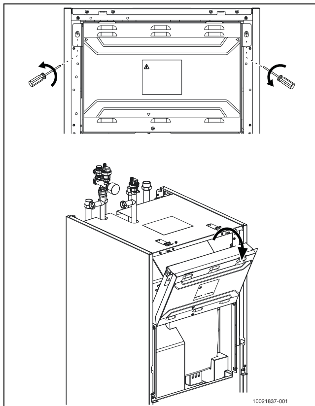
Bild 23 Klemmenkasten
