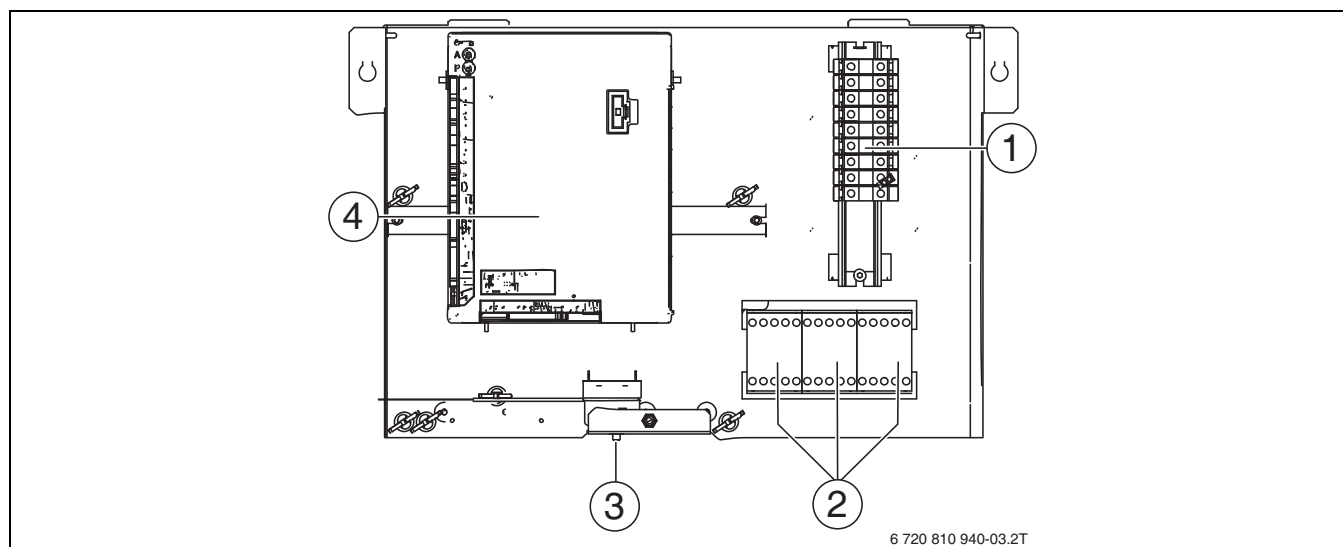
Bild 18 Klemmenkastenordnung
