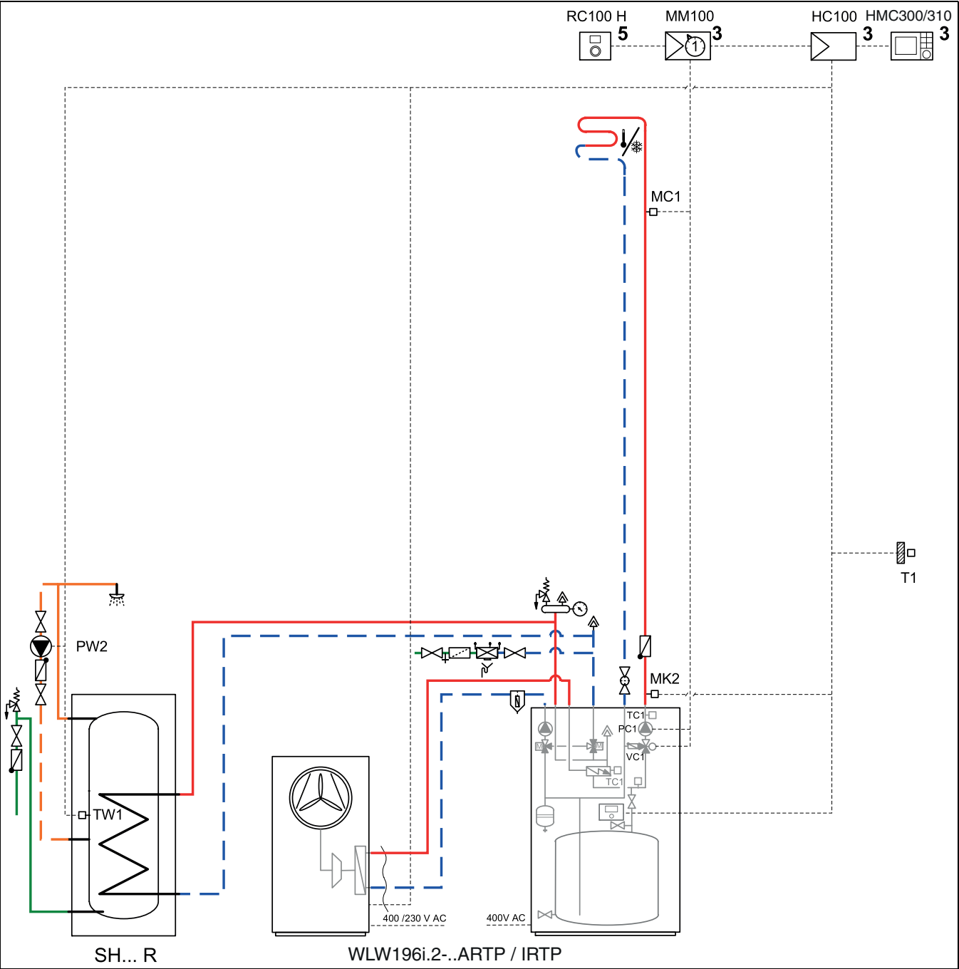
Bild 43 Wärmepumpe, Inneneinheit und gemischter Kreis
