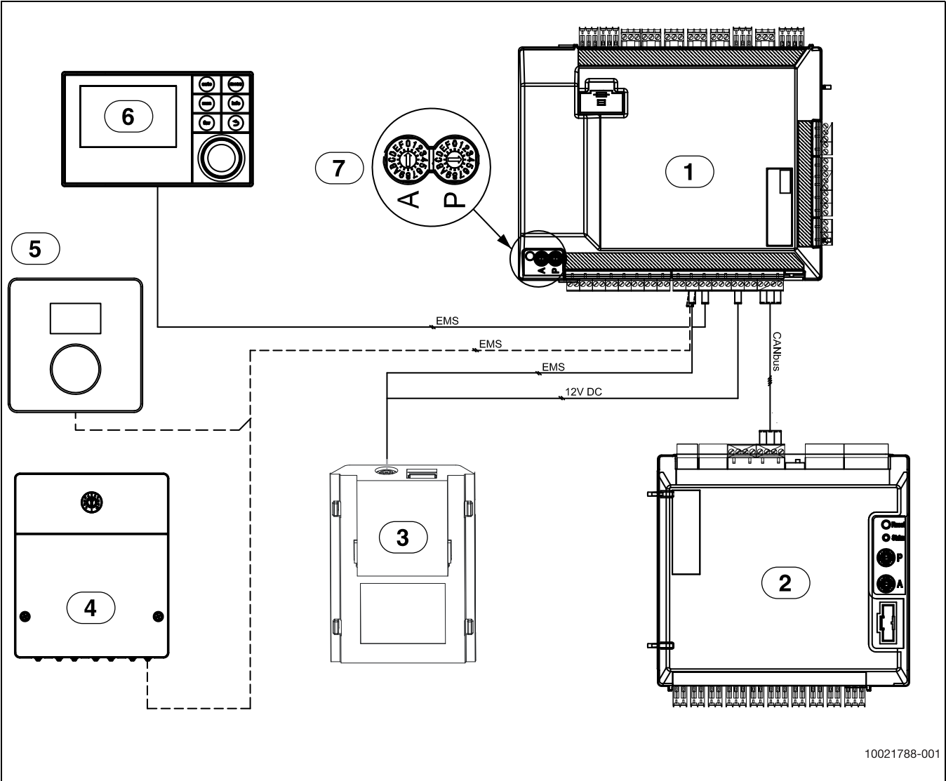
Bild 52 Schaltplan/Inneneinheit
