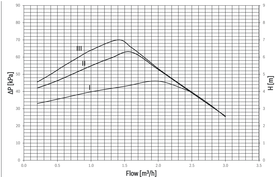
Bild 40 Restförderhöhe Heizkreispumpe für den Anschluss an den ungemischten Heizkreis für PC1 im Betrieb mit proportionalem Druck
