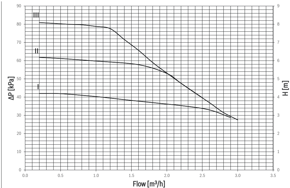
Bild 41 Restförderhöhe Heizkreispumpe für den Anschluss an den ungemischten Heizkreis für PC1 im Betrieb mit konstantem Druck
