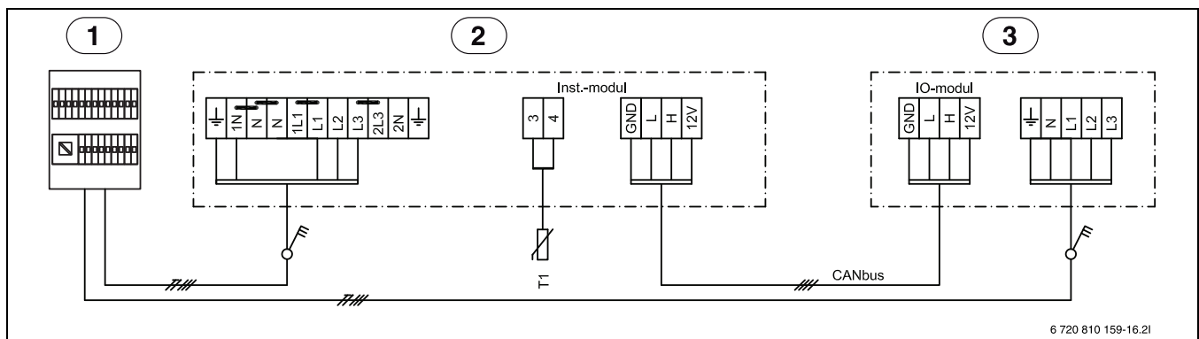
Bild 47 Schaltplan 3 N~
