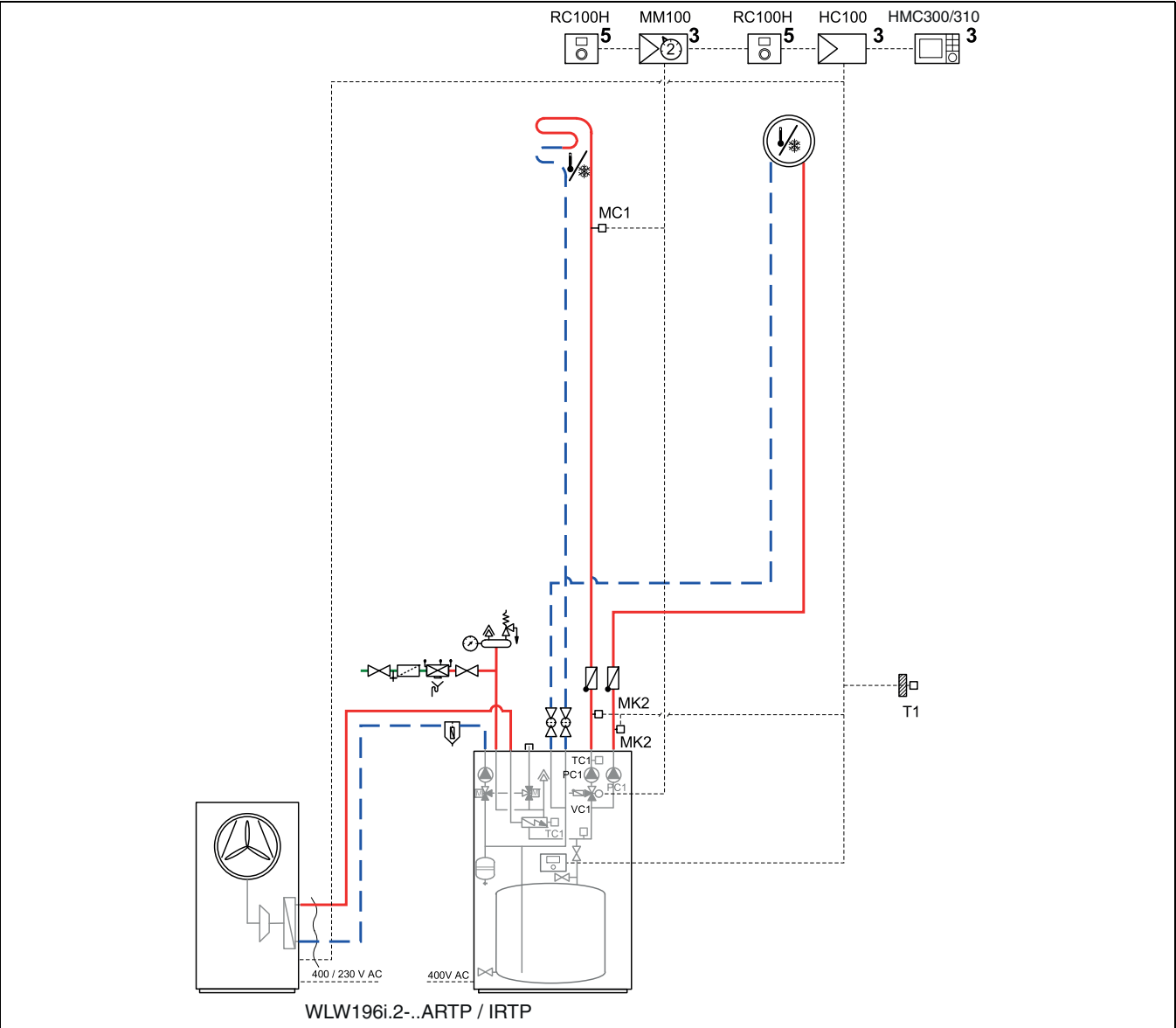
Bild 45 Wärmepumpe, Inneneinheit mit einem gemischten und einem ungemischten Kreis ohne WW
