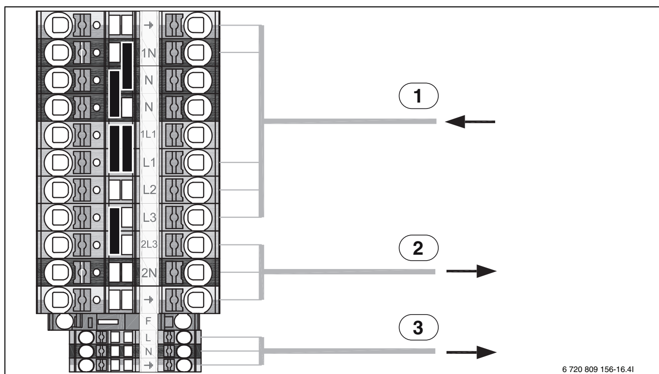
Bild 19 Klemmenbelegung im Klemmenkasten
