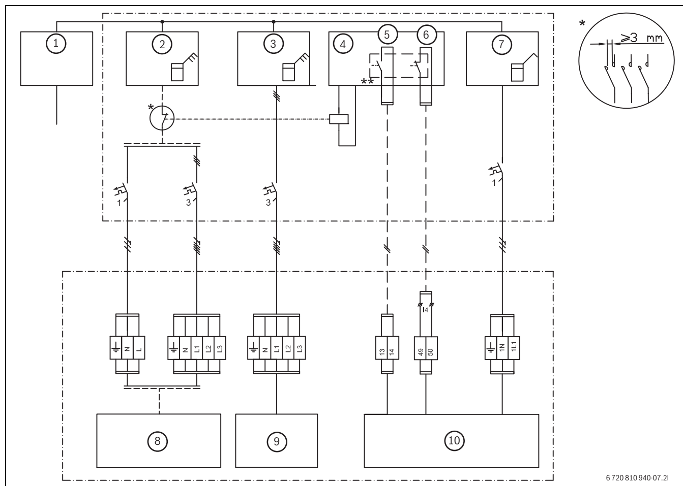
Bild 37 EVU Typ 2
