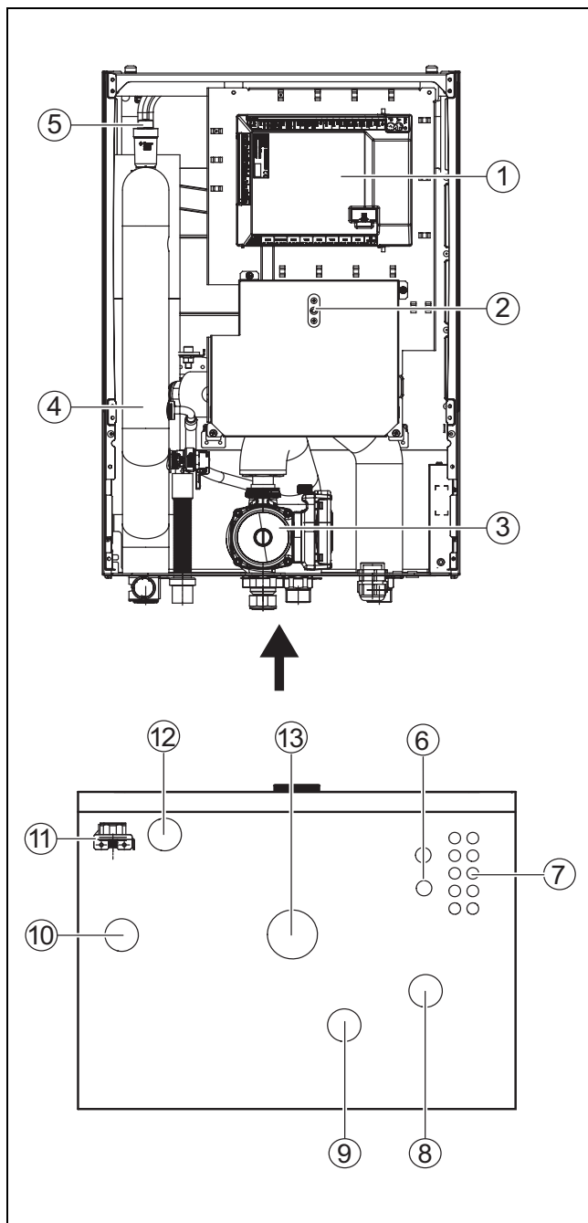
Bild 2 Bestandteile und Rohranschlüsse der Inneneinheit mit Zuheizung
