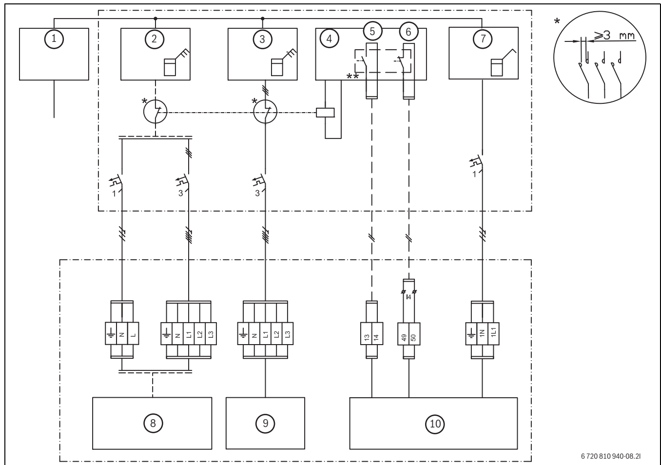
Bild 36 EVU Typ 1
