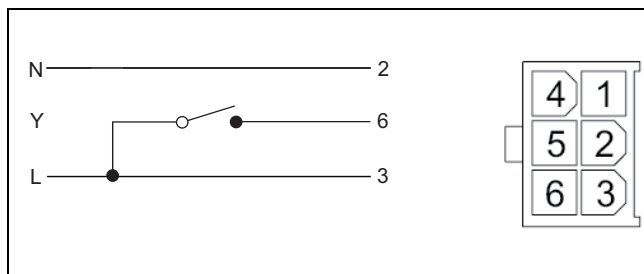
Bild 22 Molex-Stecker
