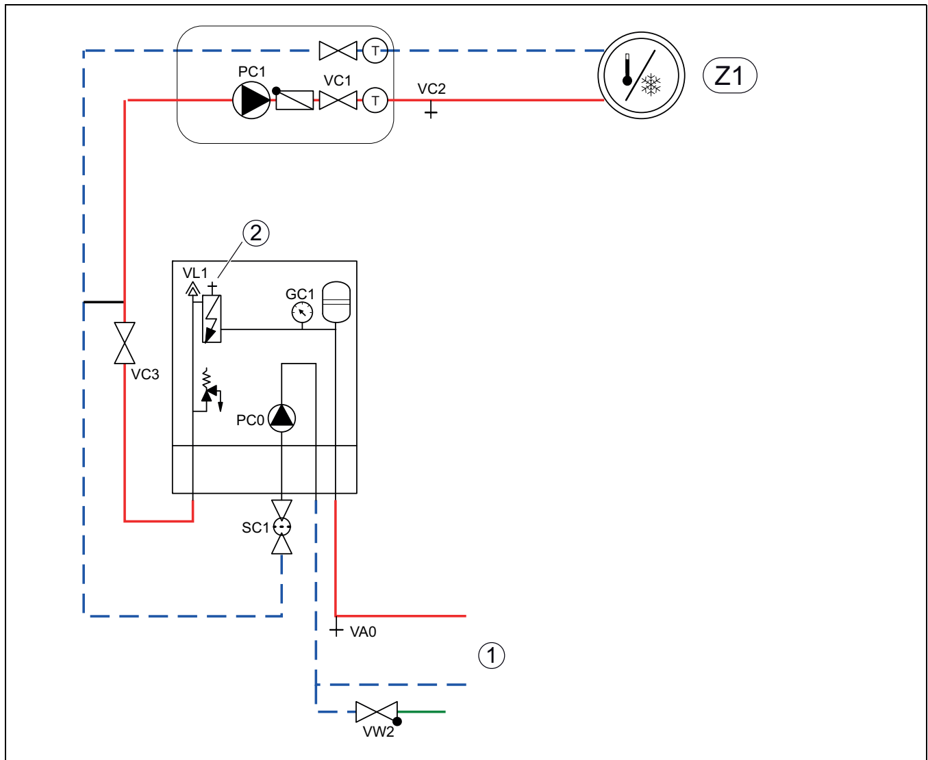
Bild 14 Inneneinheit mit integriertem elektrischen Zuheizer und Heizsystem
