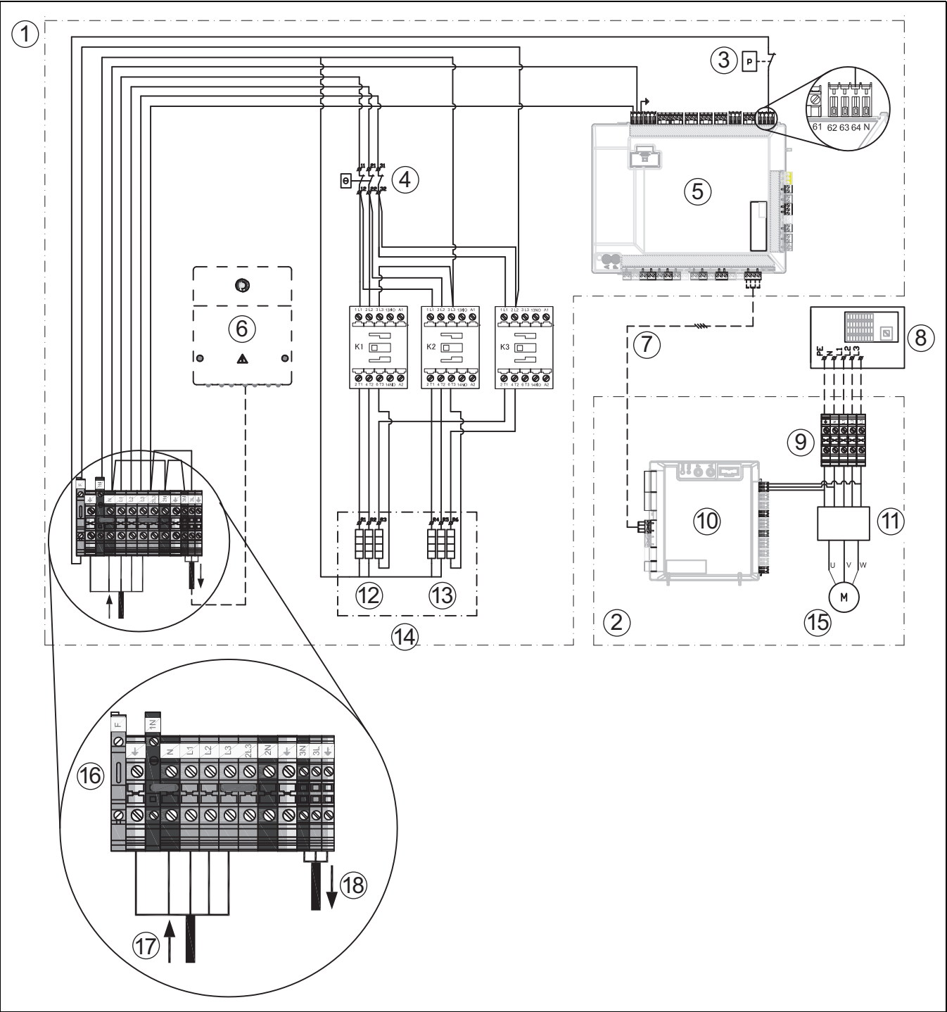
Bild 31 Wärmepumpe (Drehstrom) mit integriertem elektrischen Zuheizter (Drehstrom)
