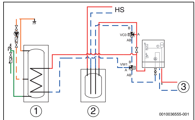
Bild 24 Puffer, VC0-Bypassventil
