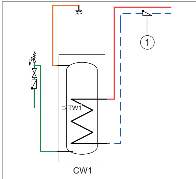
Bild 18 Warmwasserspeicher
