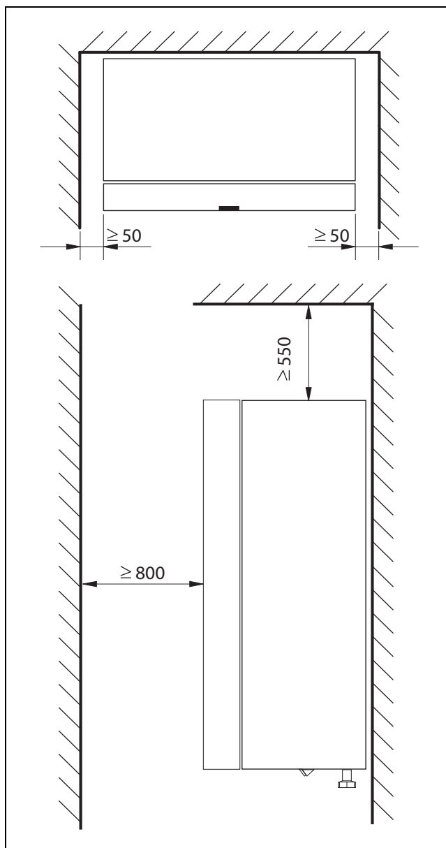
Bild 3 Mindestabstand (mm)
