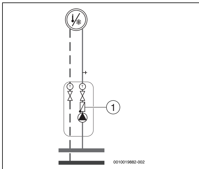
Bild 27 Heizkreis
