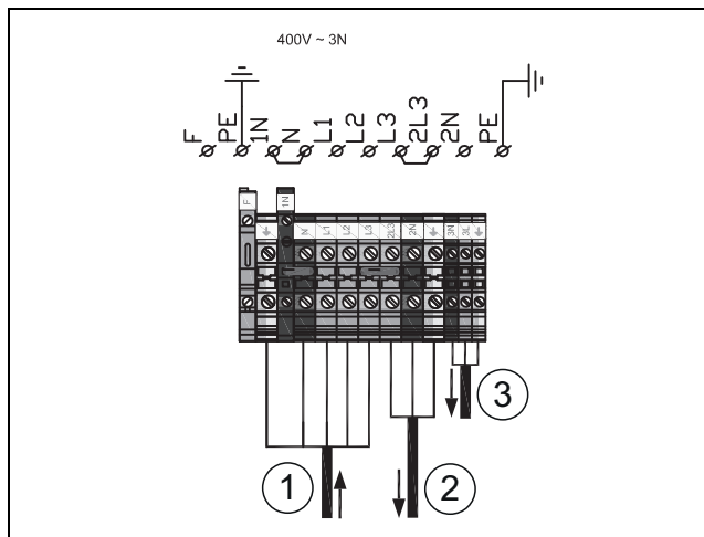
Bild 11 Elektrischer Standardanschluss bei integriertem elektrischen Zuheizter
