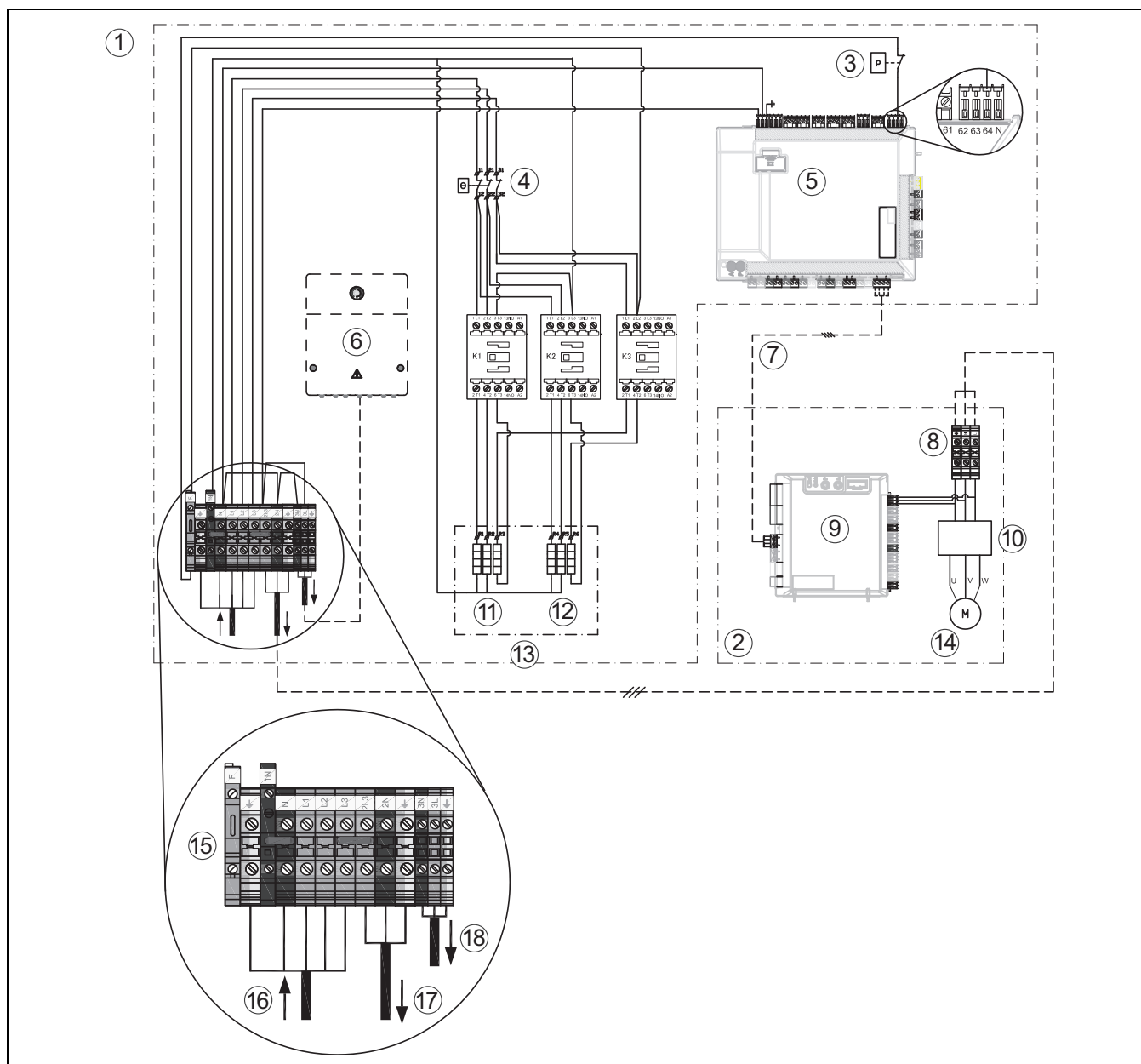
Bild 30 Einphasige Wärmepumpe mit integriertem elektrischen Zuheizer (Dreistrom)
