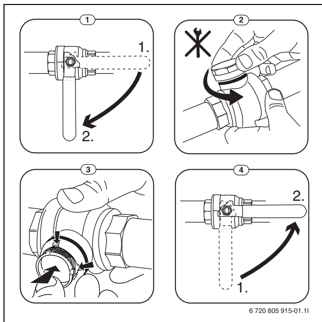
Bild 16 Siebreinigung
