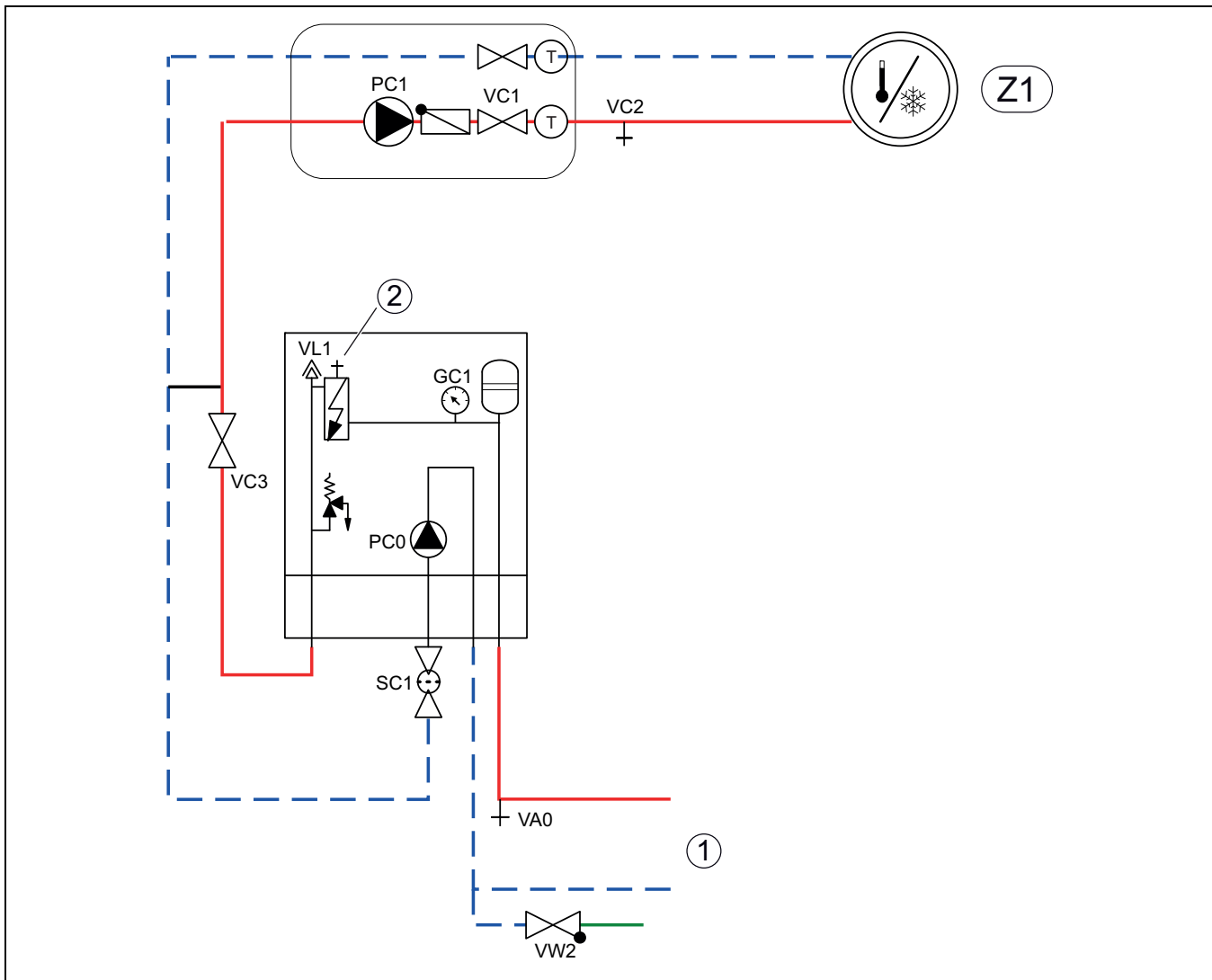
Bild 7 Inneneinheit mit integriertem elektrischen Zuheizer und Heizsystem
