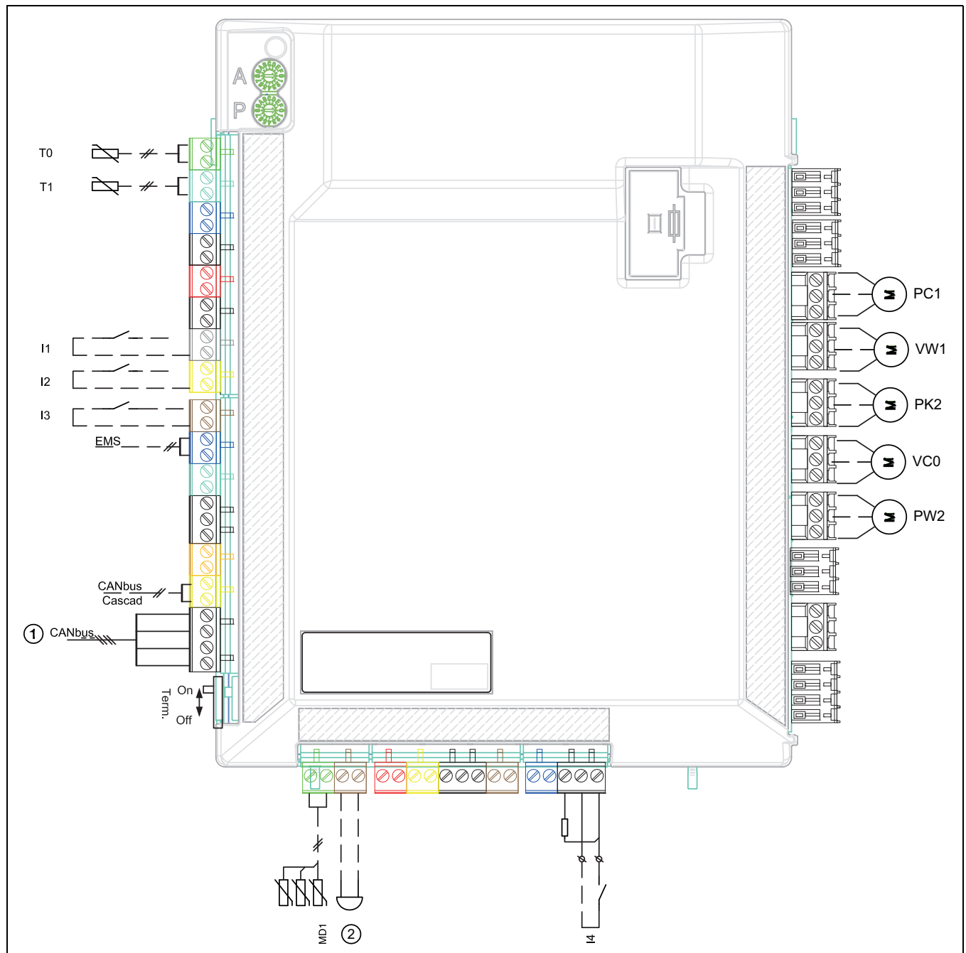
Bild 12 Anschlüsse Installationsmodul
