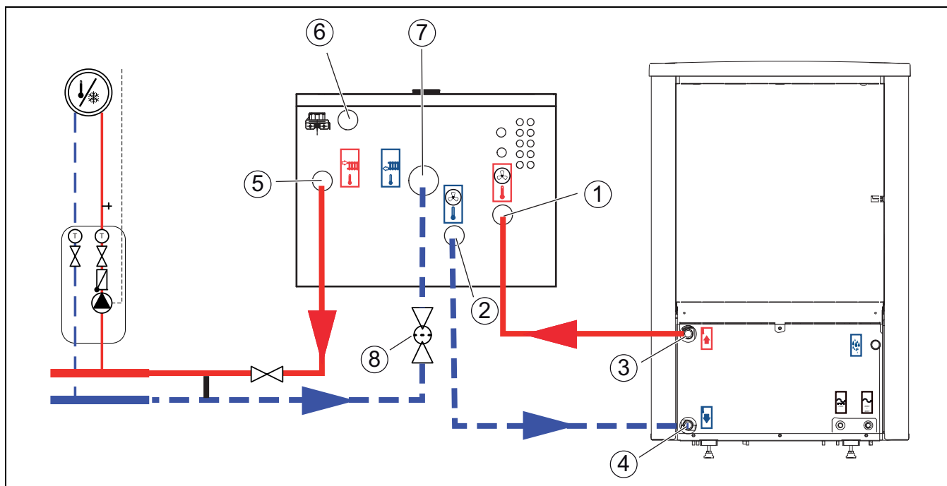
Bild 6 Anschluss des Inneneinheits mit elektrischem Zuheizer an Wärmepumpe und Heizungsanlage
