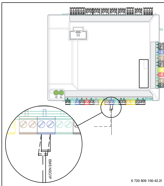
Bild 17 EMS-Anschluss am Installationsmodul
