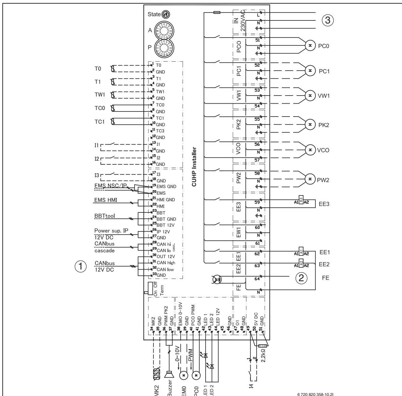
Bild 32 Schaltplan Installationsmodul mit integriertem elektrischen Zuheizer
