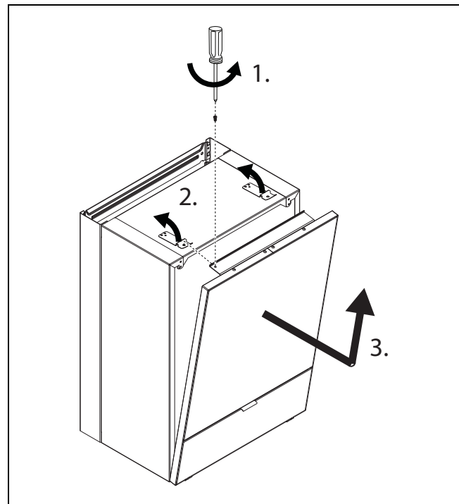
Bild 5 Frontplatte abnehmen
