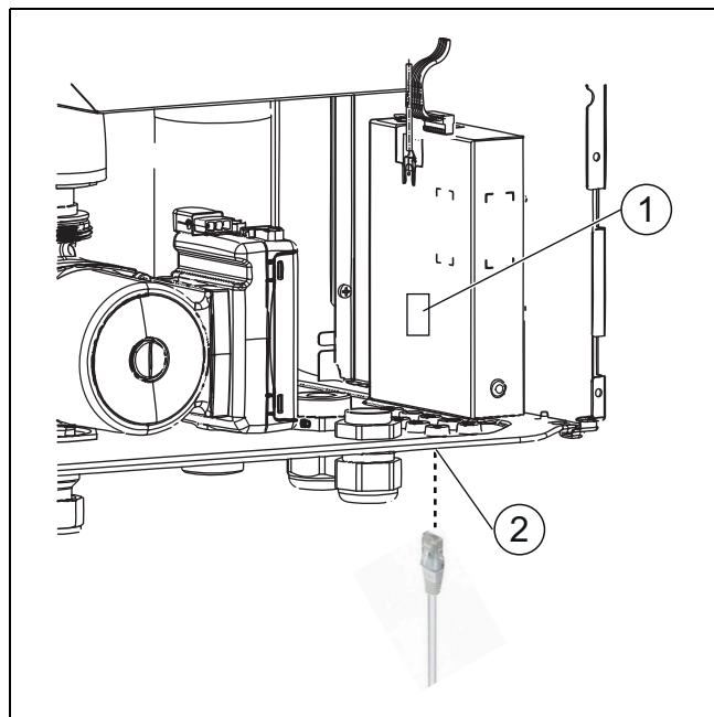
Bild 25 IP-Modul
