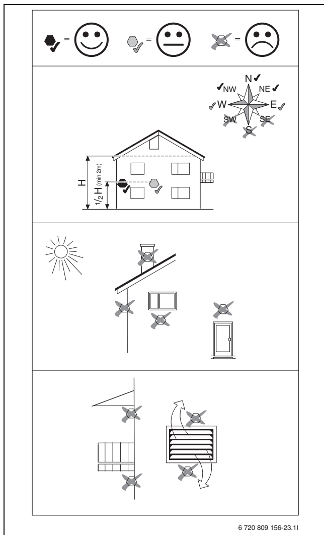
Bild 9 Platzierung des Außentemperaturfühlers
