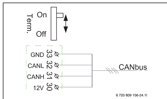
Bild 8 CAN-BUS-Terminierung
