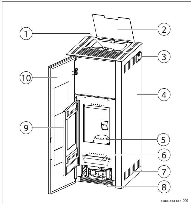
Bild 3 Produktübersicht
