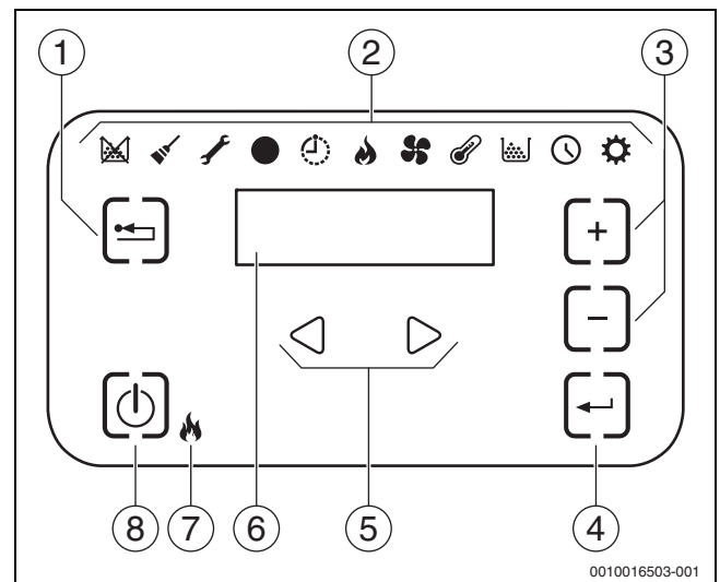
Bild 8 Bedienfeld
