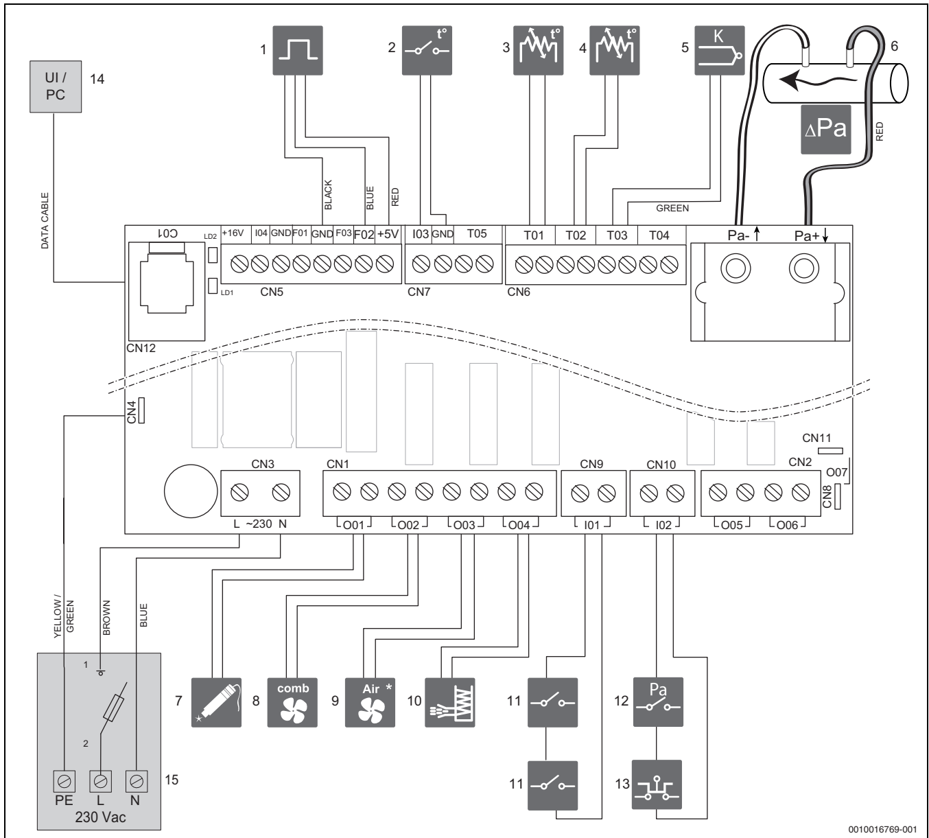
Bild 10 Anschlussplan
