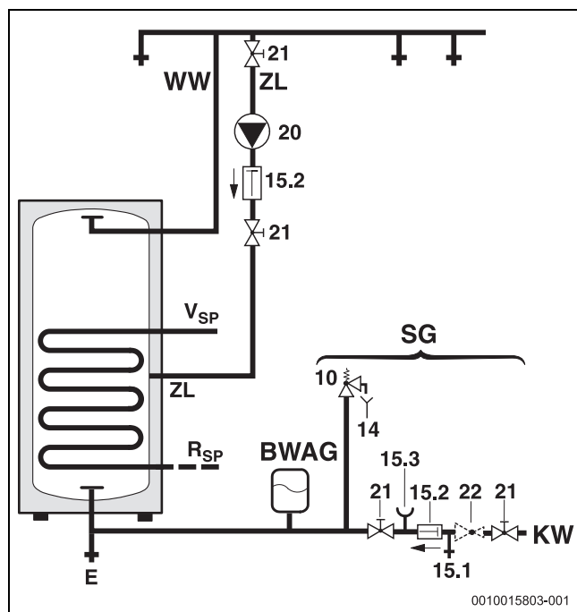
Afb. 4 Aansluitschema drinkwaterzijde
