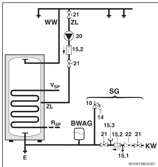
Bild 1 Trinkwasserseitiges Anschluss-Schema
