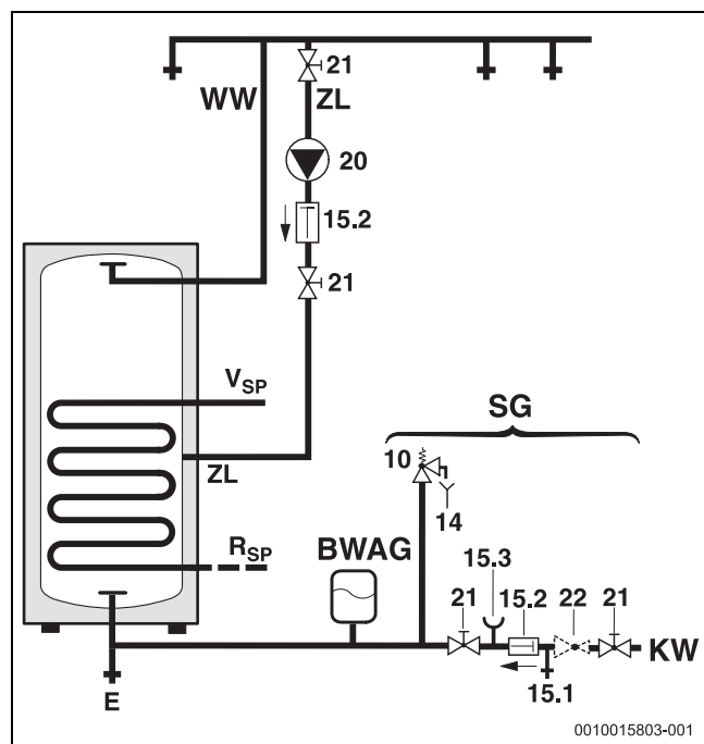
Sl.6 Shema prikliučka na strani pitke vode
