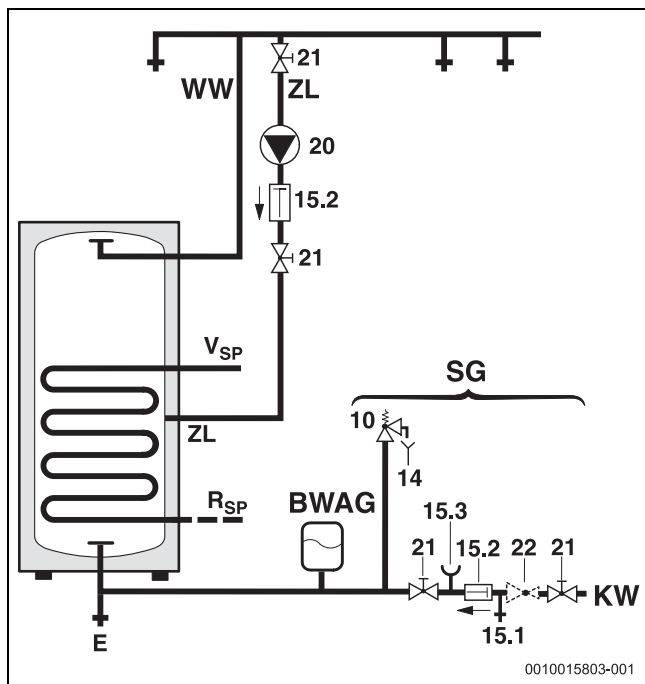
Joon. 3 Tarbeveepoole ühendusskeem
