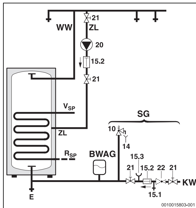
Fig. 5 Schéma de raccordement côté eau chaude sanitaire
