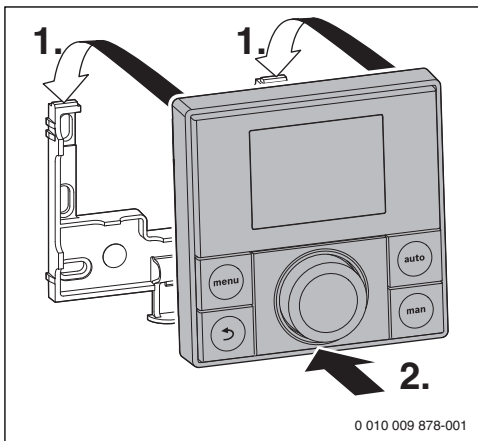
Bild 5 Bedieneinheit einhängen
