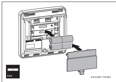
Bild 4 Batterien einsetzen
