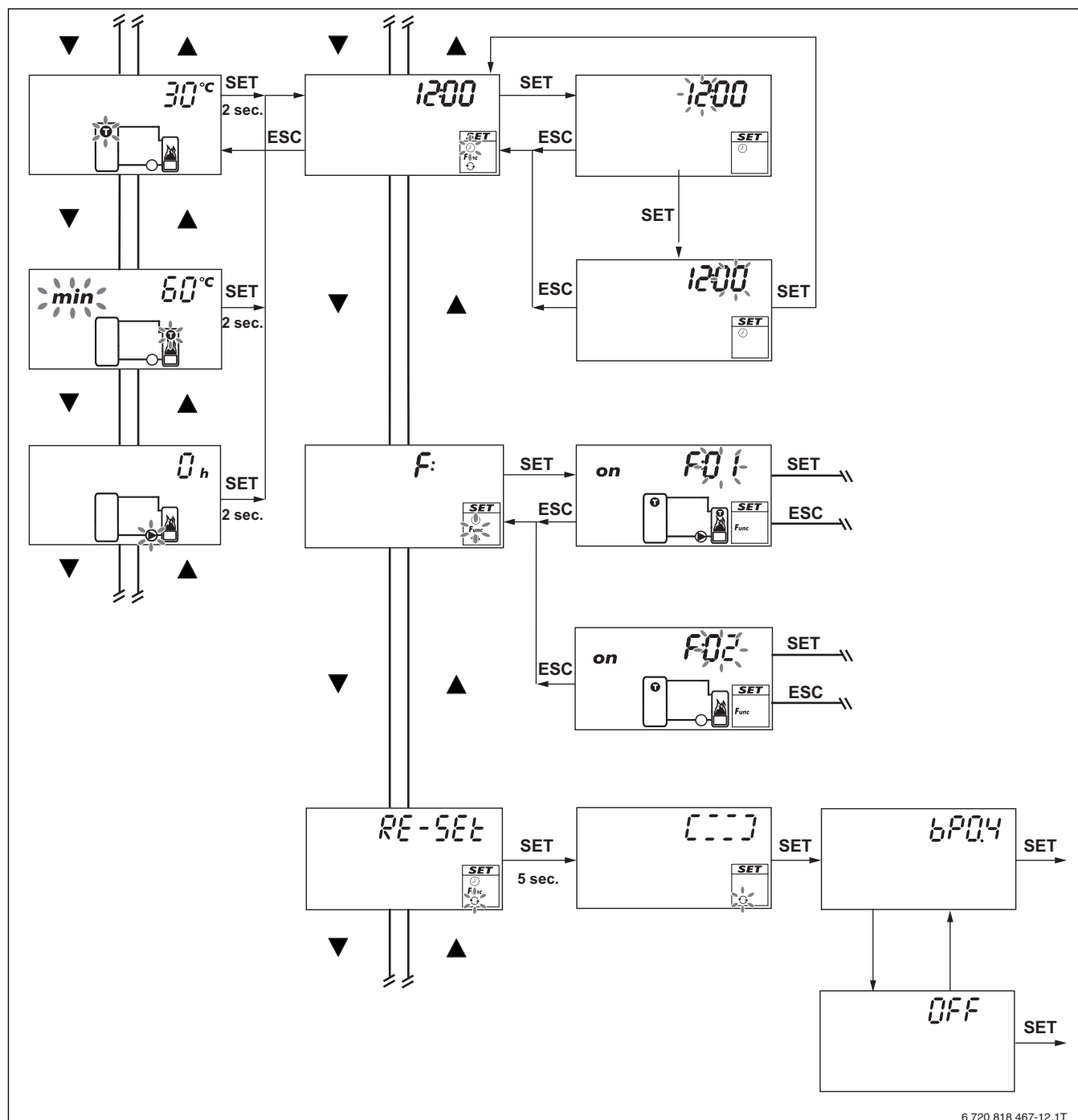
Bild 27 Funktionsschema Fachmannebene
