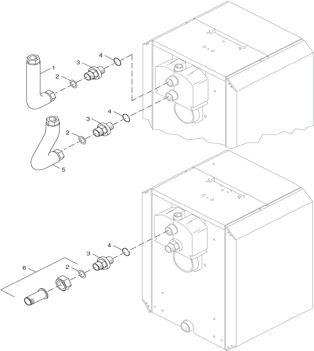
8738892023.aa.RO-Anschlussrohrgruppe KAS10
