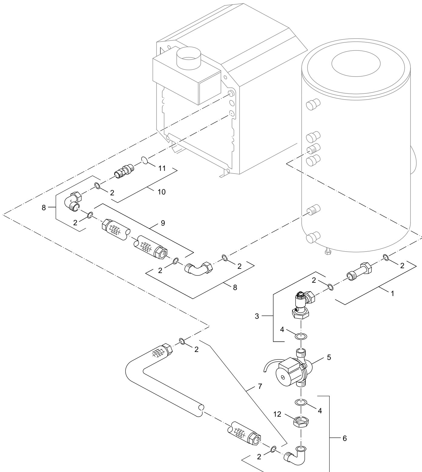
99900122.aa.RS-Kessel-Speicherverrohrung G134X SU
