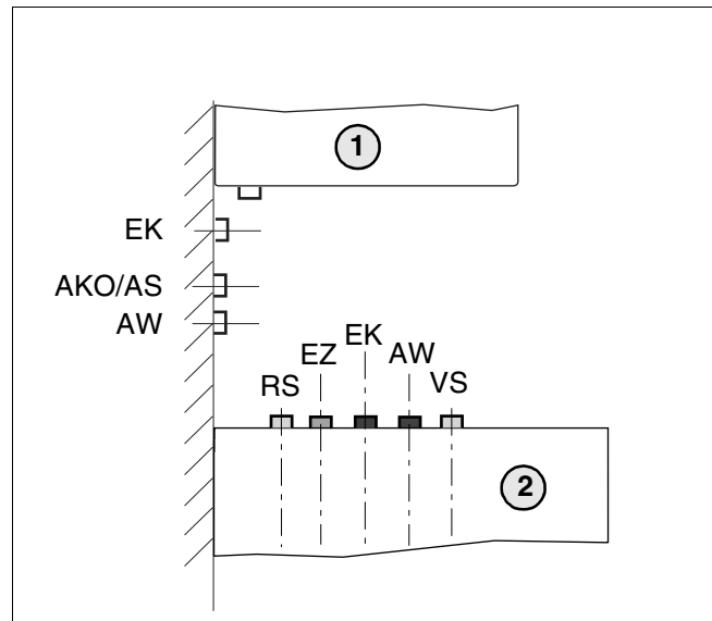
Abb. 3 Abmessungen der Hydraulikanschlüsse S135/S160, Unterputzmontage (Seitenansicht)
